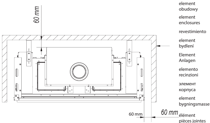
Rys. 3. Minimalne odległości wkładu gazowego od niepalnych elementów obudowy
