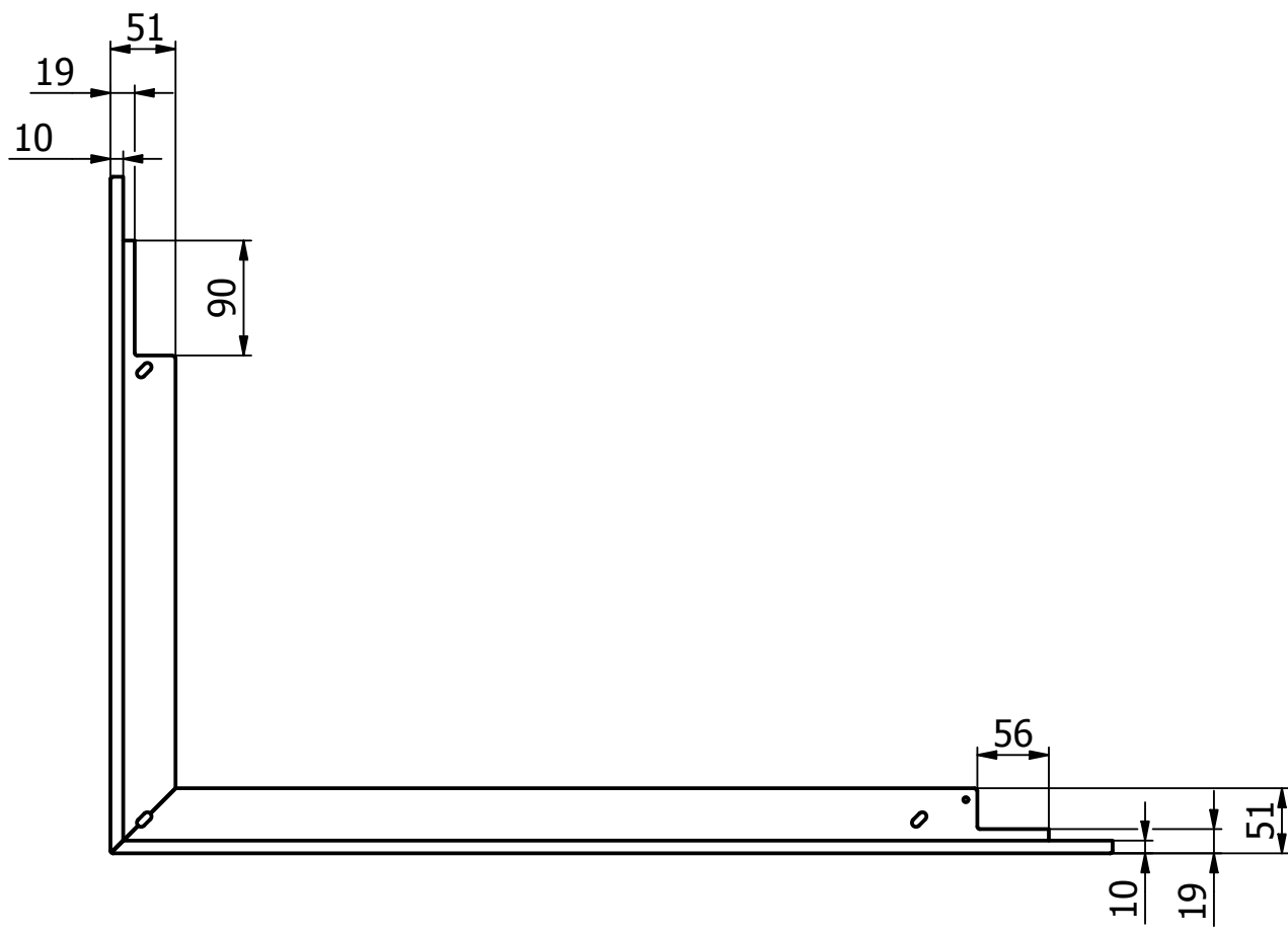
Maskownica 50 płytka
