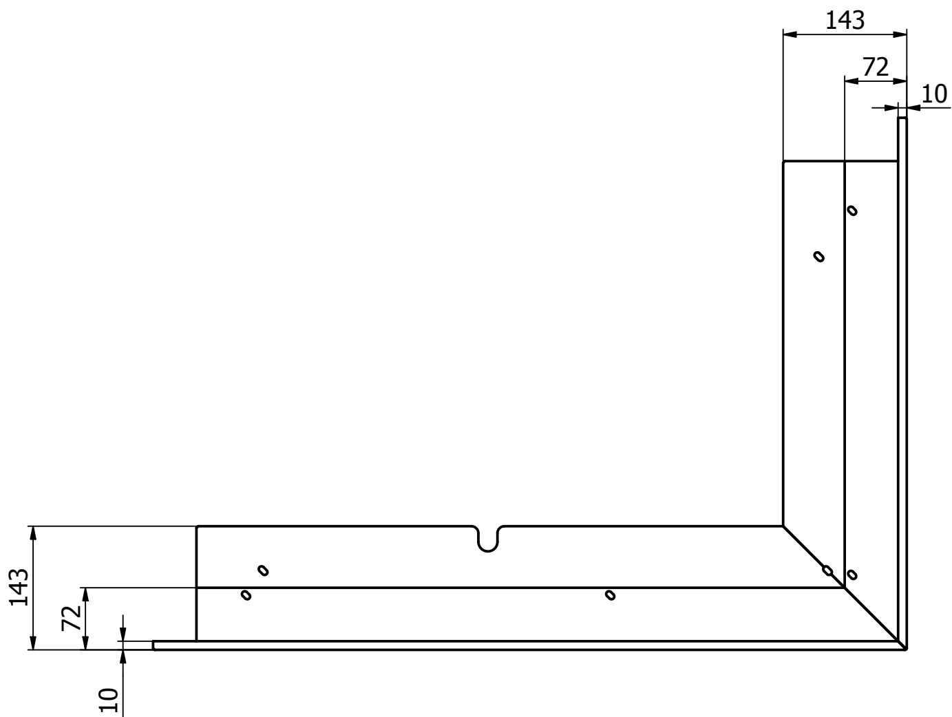
Maskownica 50 głęboka
